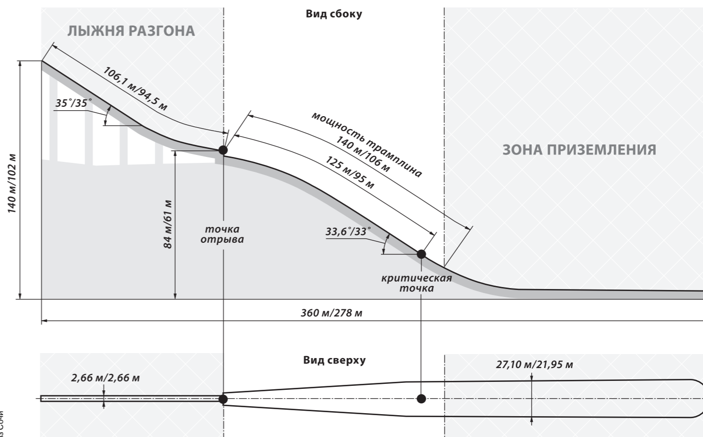
Профили обоих трамплинов практически идентичны. Все размеры указаны по схеме: К-125/К-95.
